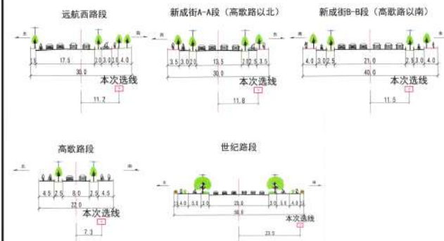
道路管线规划断面图
