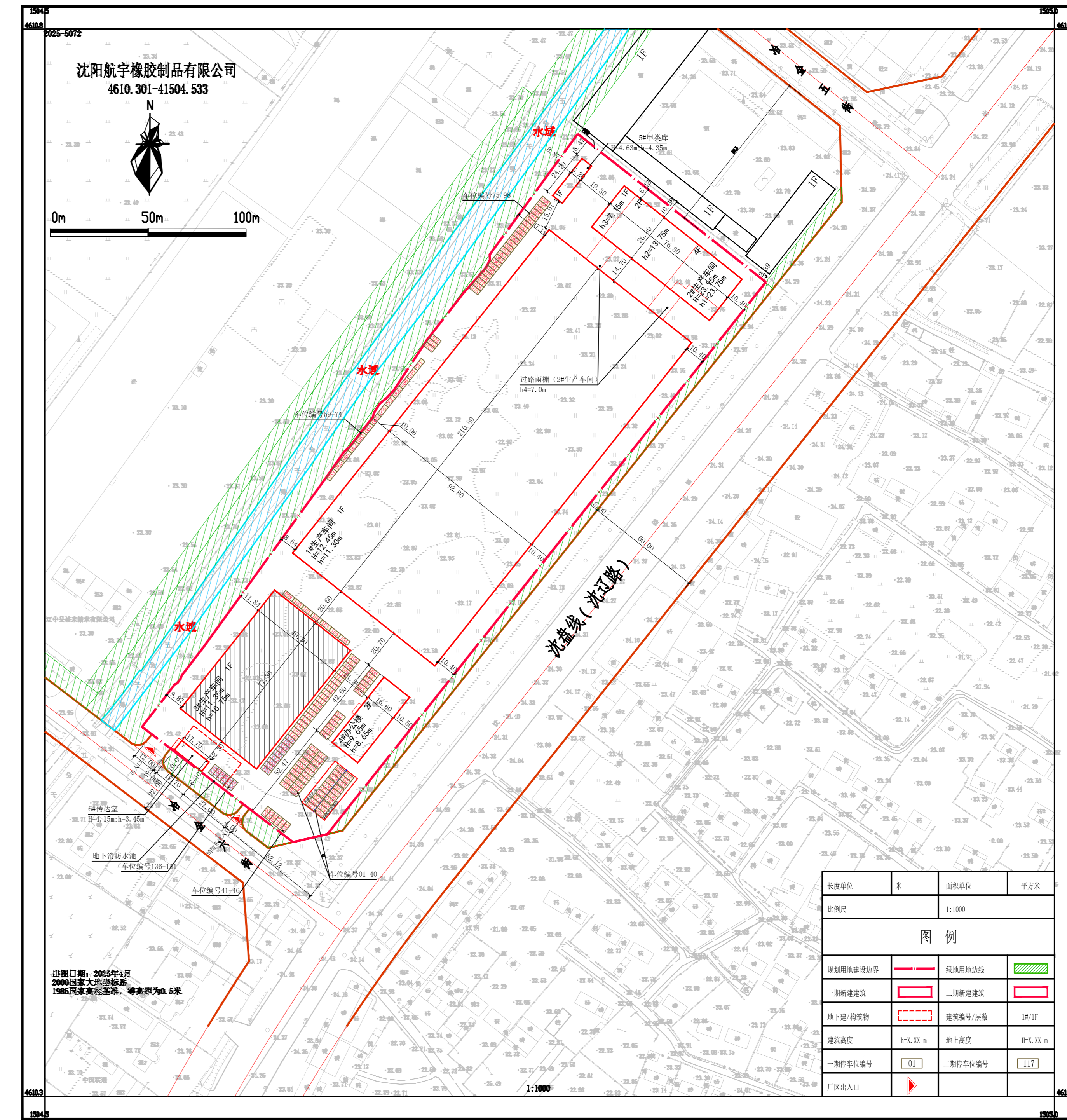
变更后总平面图
