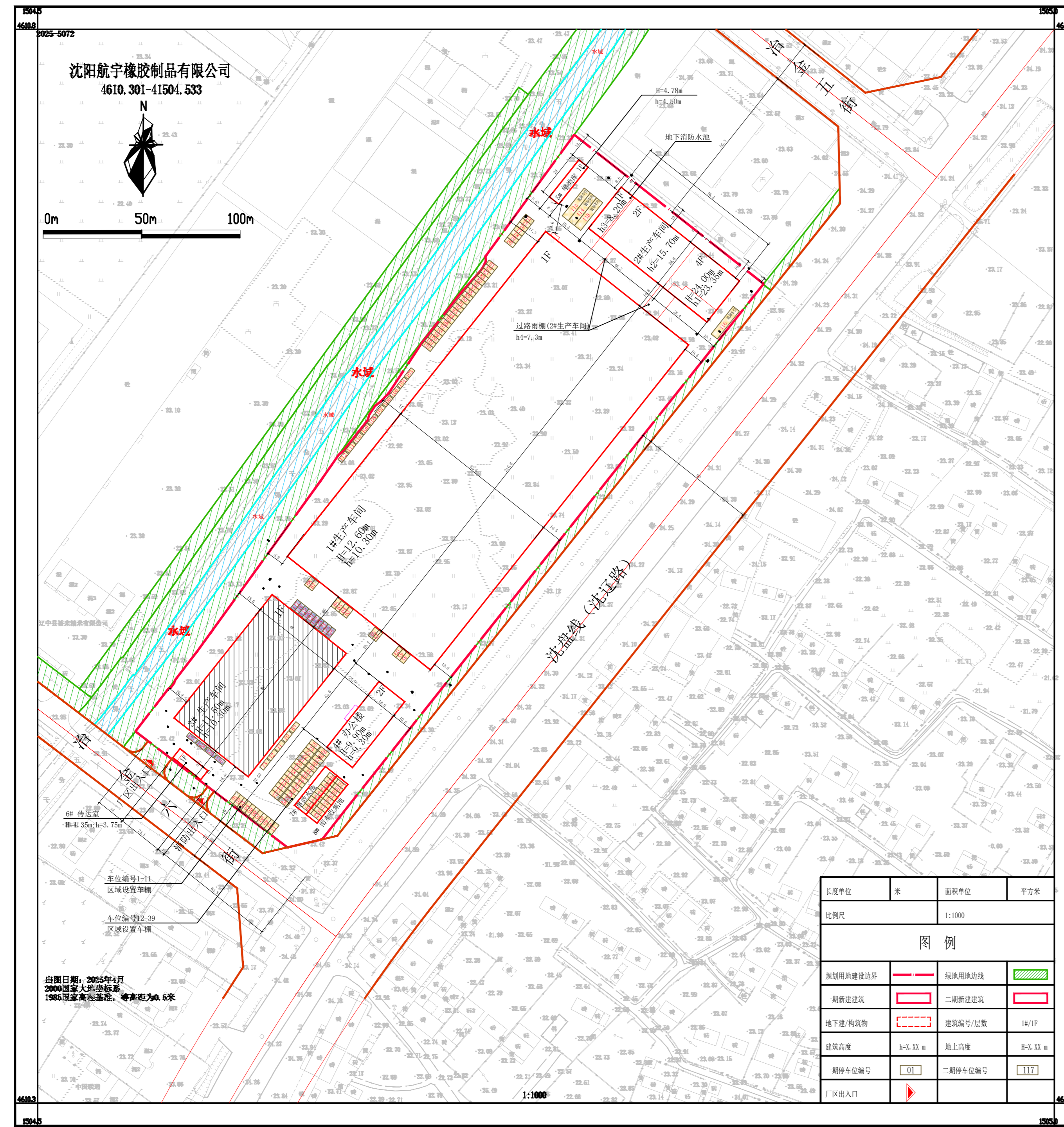
变更前总平面图
