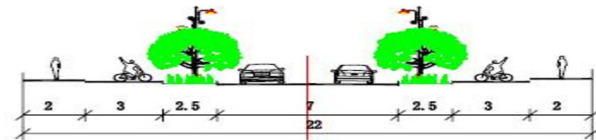
3号路西段道路规划横断面
