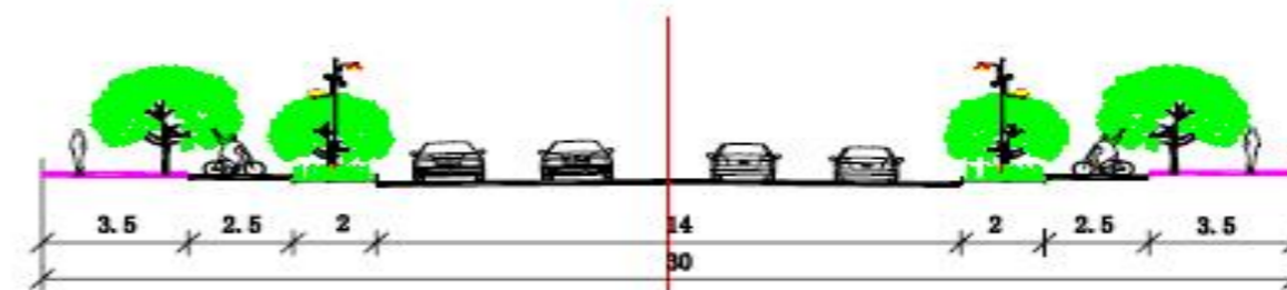
2号路西段道路规划横断面
