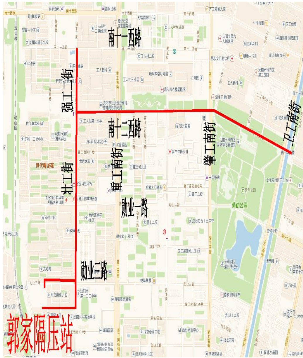
规划线位方案平面图
