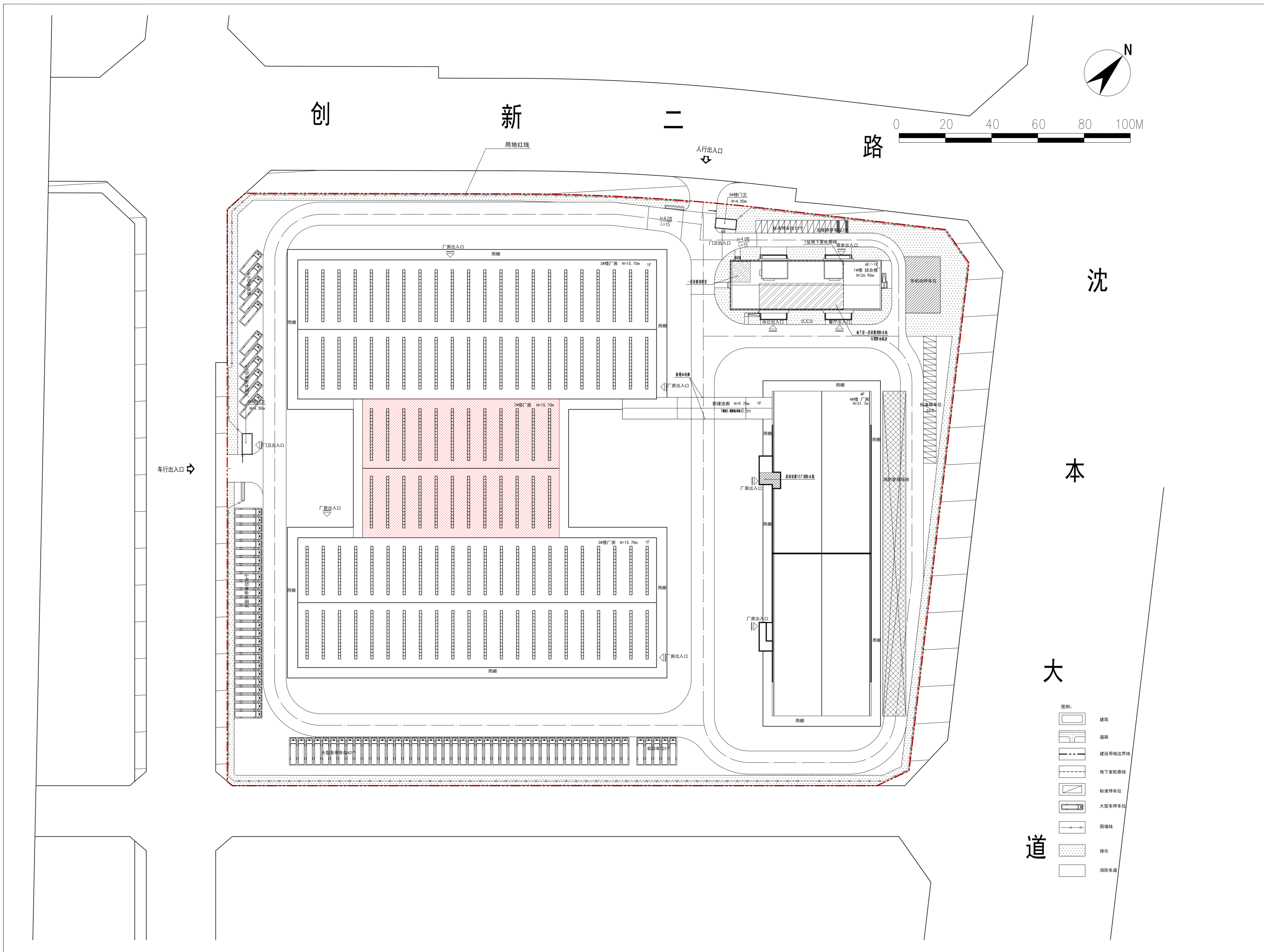
规划设计方案总平面图
