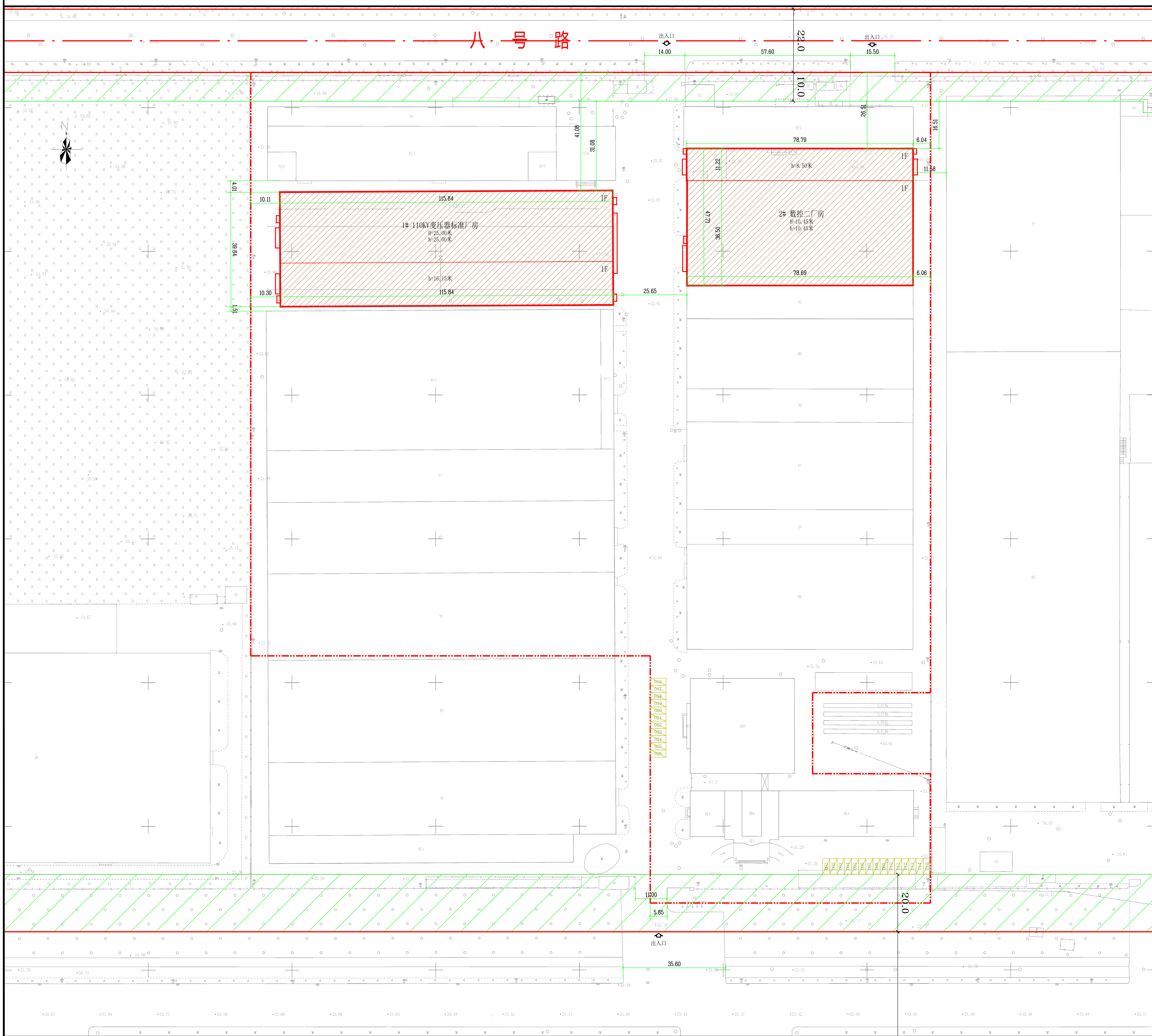
规划设计方案总平面图
