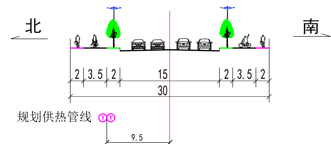
规划断面图C-C
