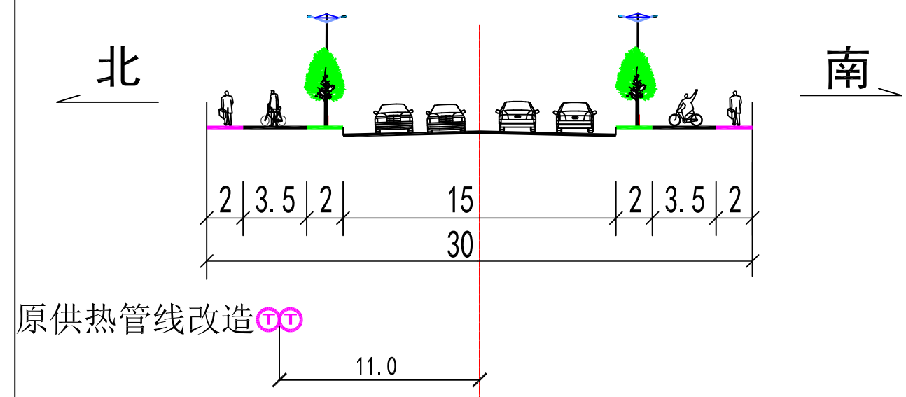
规划断面图D-D
