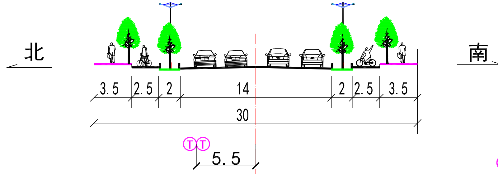
三环南三路（文溯南街东四街-文溯南街东五街）规划断面图
