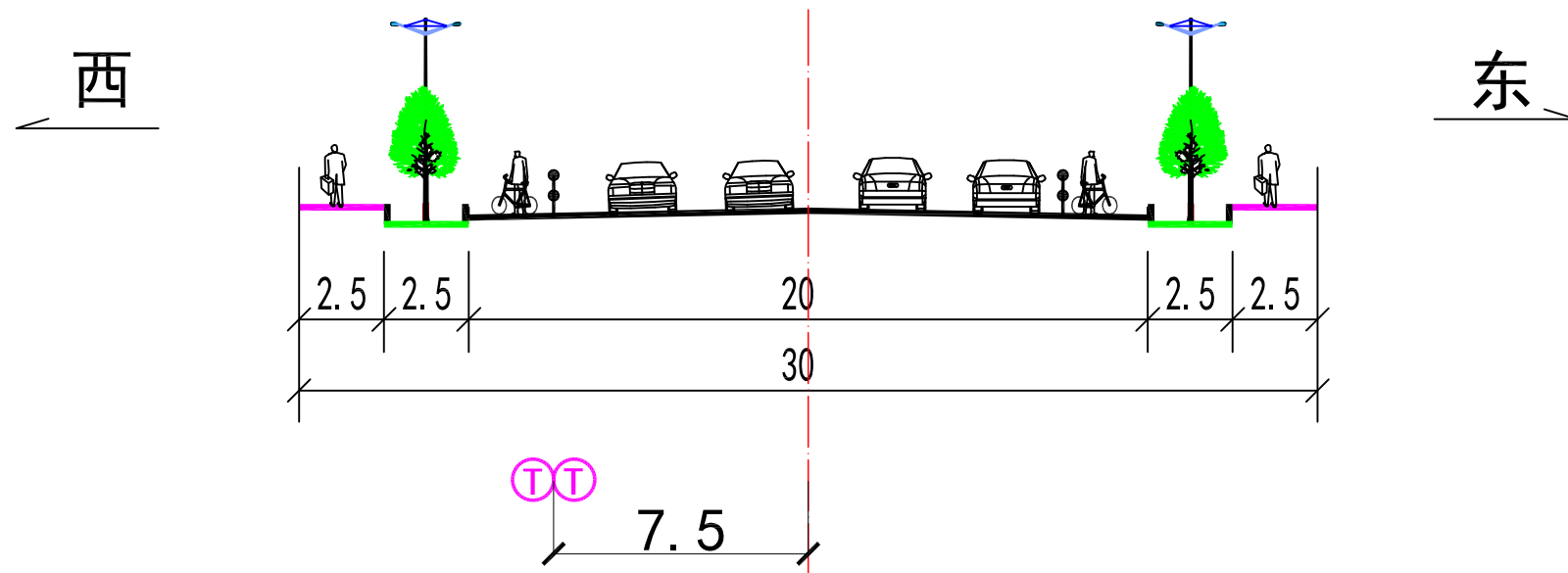
三环南三路（文溯南街东三街-文溯南街东四街）规划断面图
