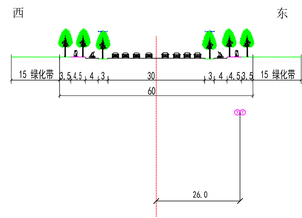
规划断面图A-A
