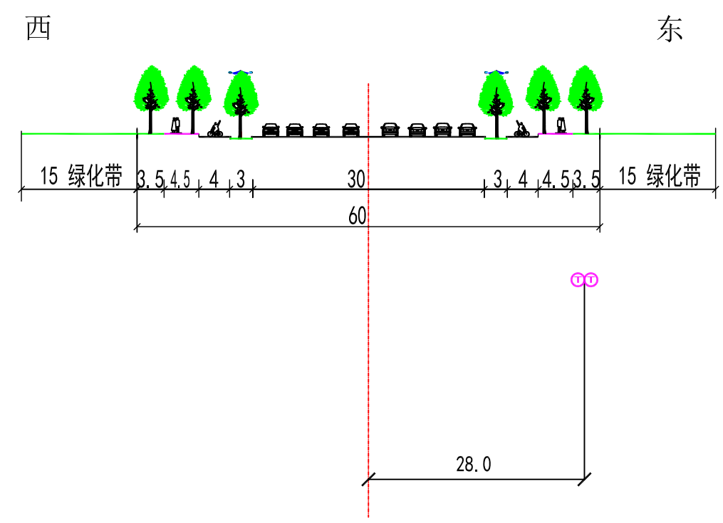
规划断面图B-B
