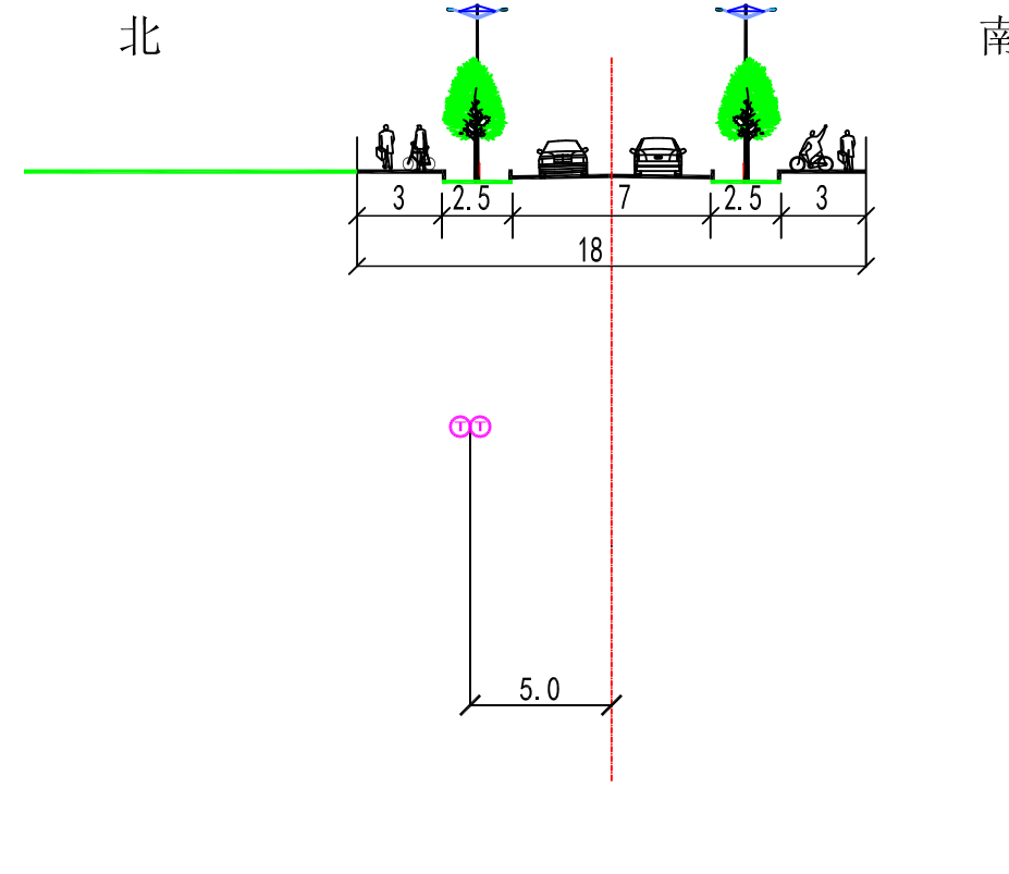
规划断面图C-C
