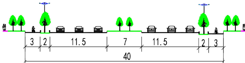
长安桥南街规划横断面
