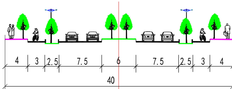
新南堤路规划横断面
